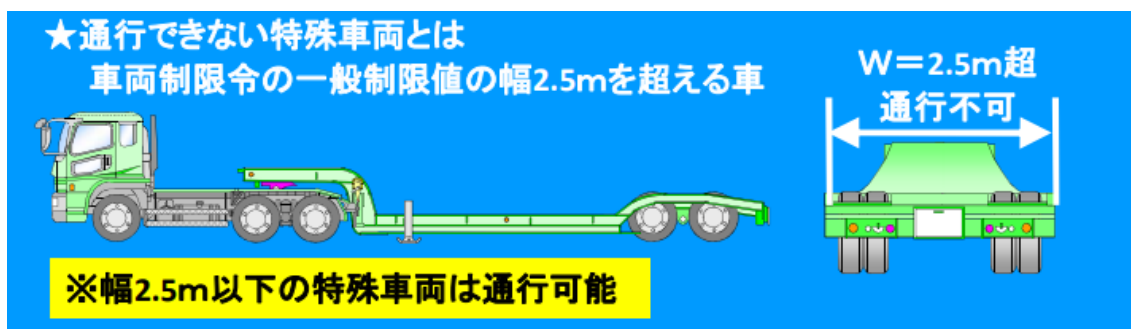
特殊車両（車幅 2.5m 超の幅広車）
